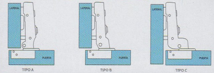
BISAGRA DE CERRADO SUAVE REF. F05C-F40 Acero niquelado
